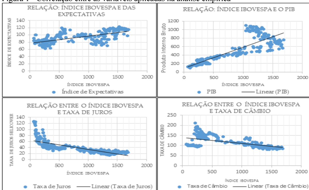
Figura 1 - Correlação entre as variáveis aplicadas na análise empírica
