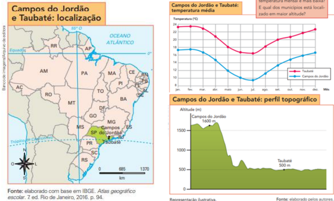
Figura 7 – Campos do Jordão e Taubaté: localização, temperatura, perfil topográfico
