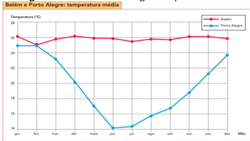
Figura 6 – Belém e Porto Alegre: temperatura média
